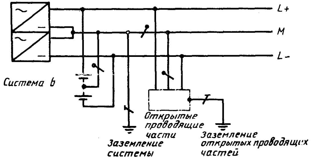
Рисунок 31J - Система TT постоянного тока
