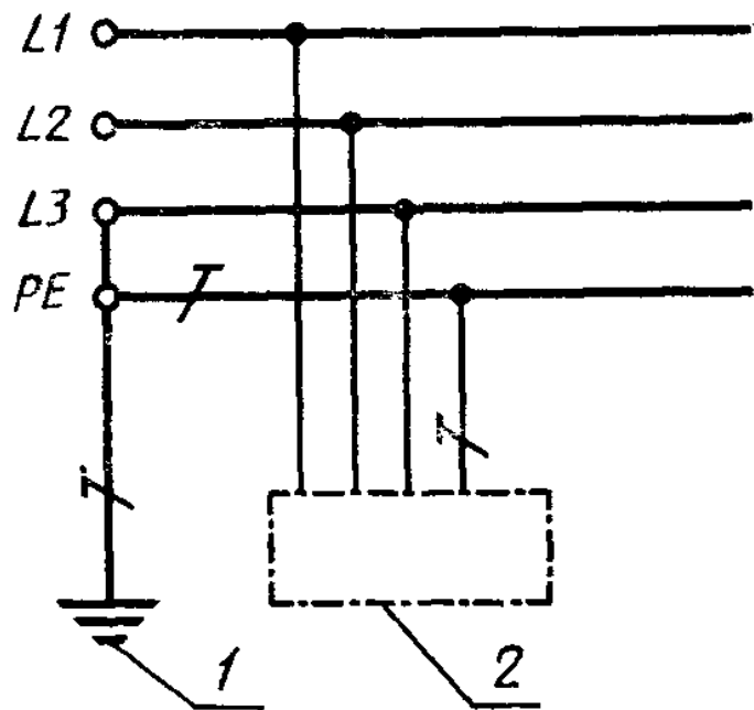
Рисунок 31А - Система TN-S (нулевой рабочий и нулевой защитный проводники работают отдельно)
