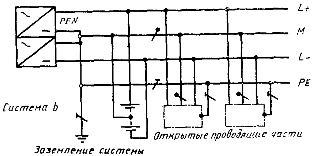
Рисунок 31F - Система TN-S постоянного тока
