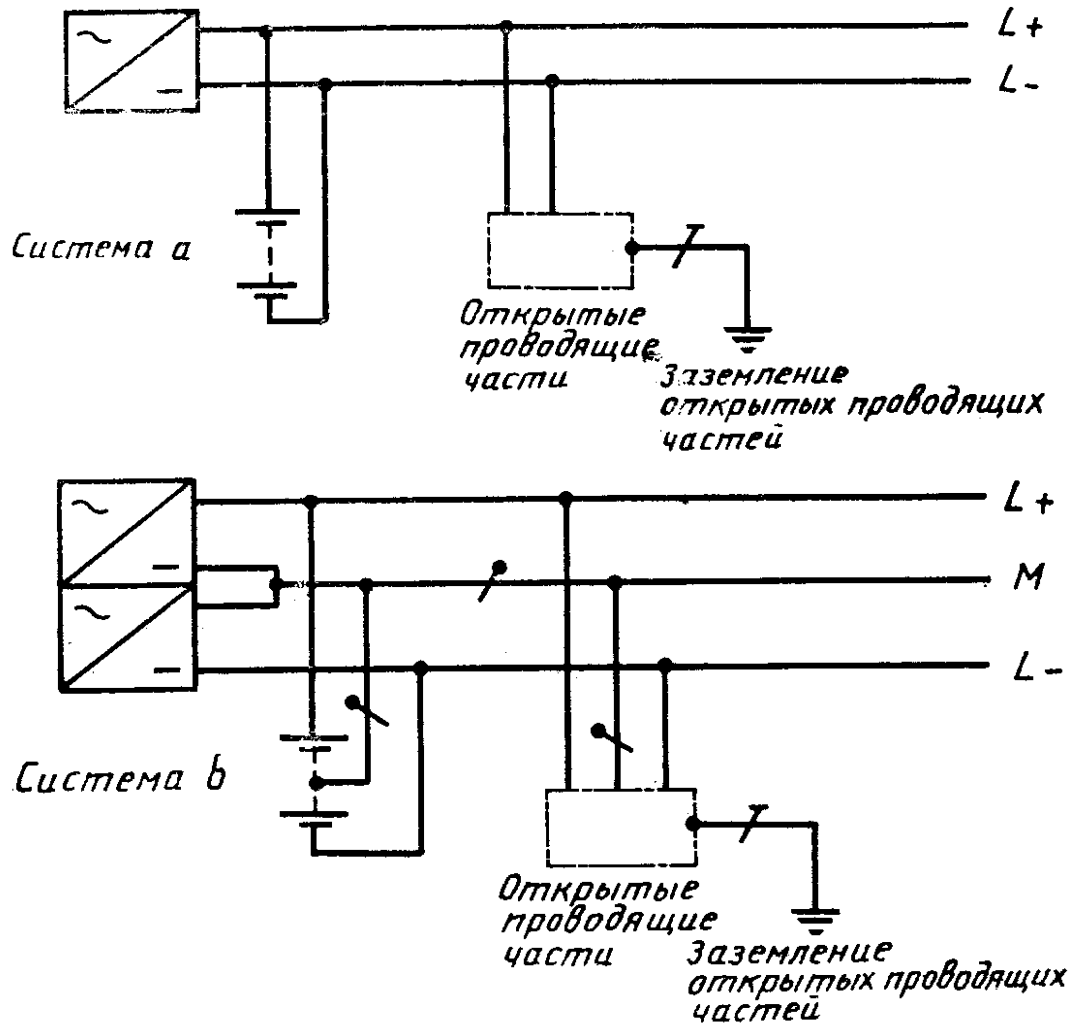
Рисунок 31К - Система IT постоянного тока
